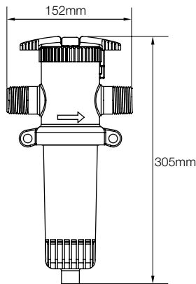
Dimensions filtres en 1" et 3/4"
