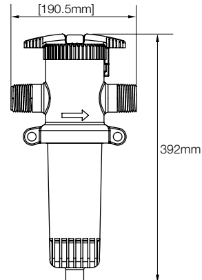
Dimensions filtre en 1.5"
