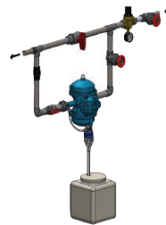
Instalación bypass
